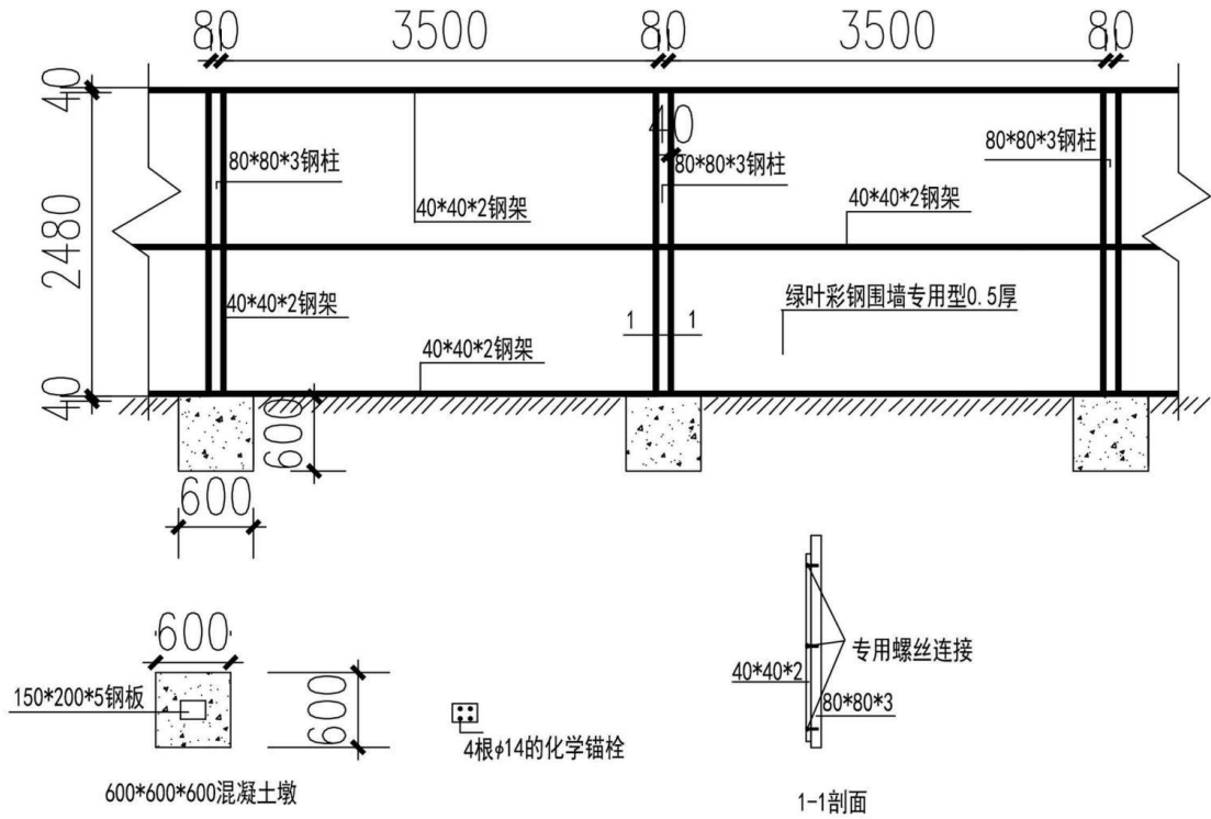
围挡施工图
