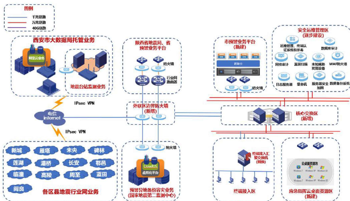
图 预警专网云数据中心改造规划设计
